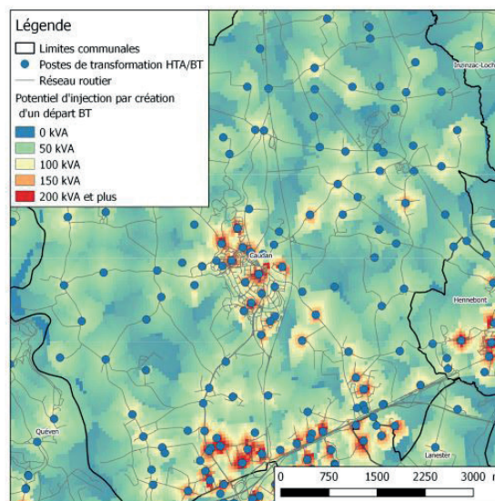
Illustration des potentiels d'injection, des postes de transformation et du réseau routier
