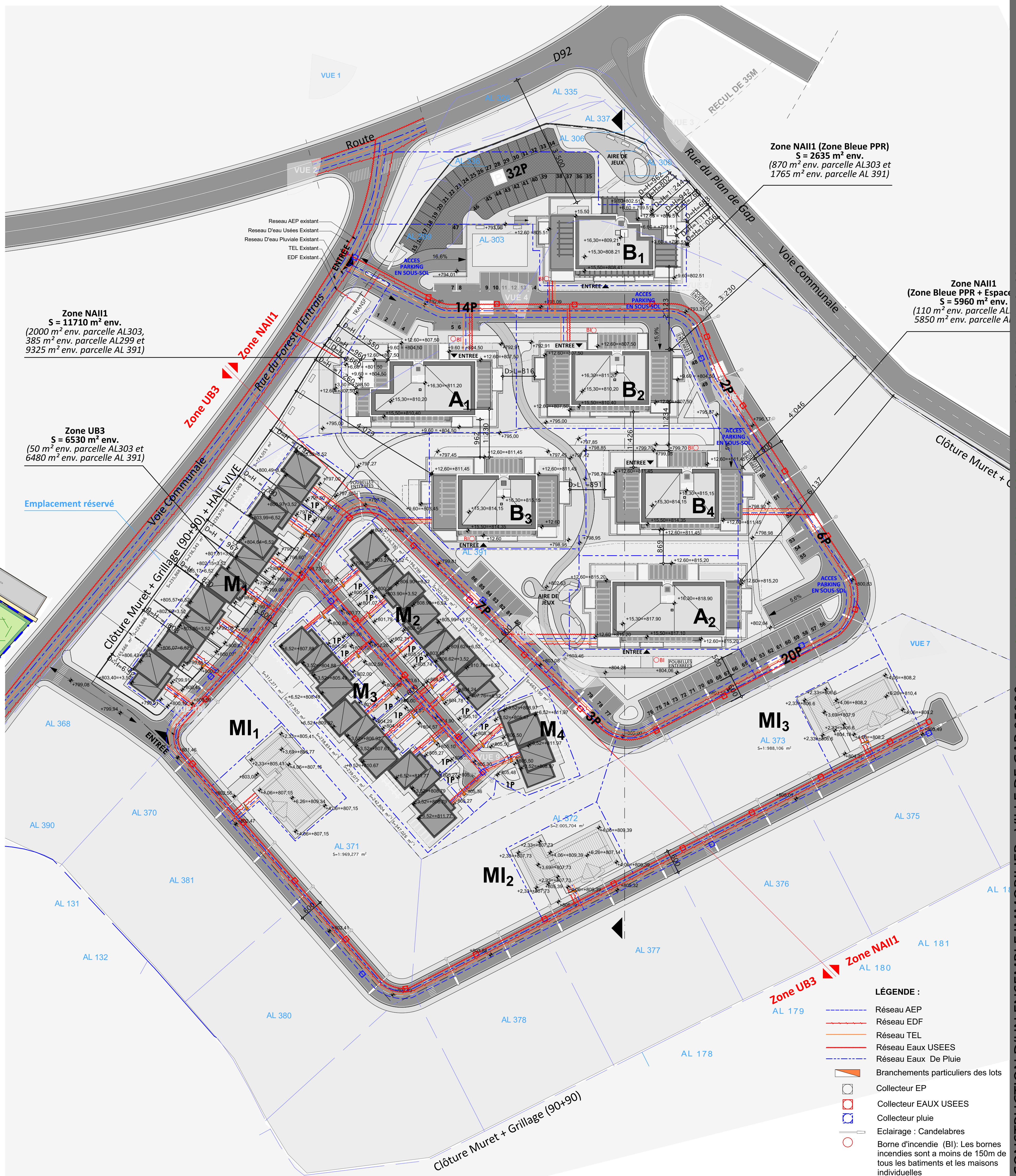
PC2: PLAN DE MASSE RESEAUX 1:500
