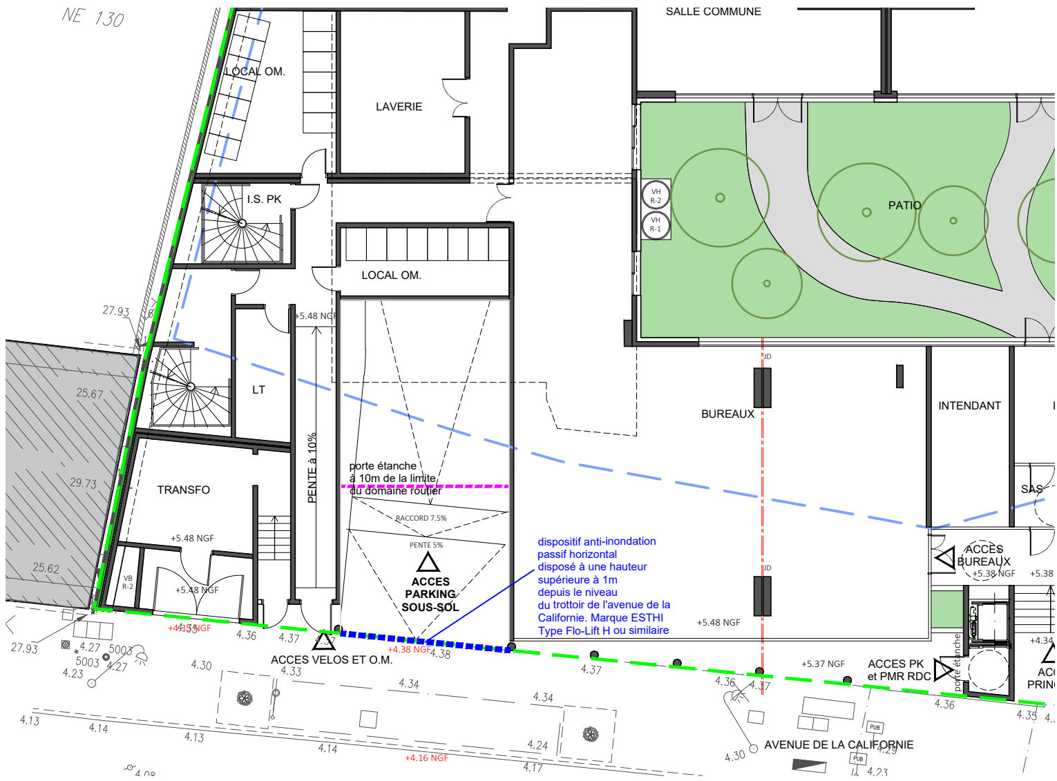
Extrait Plan de RDC 1-200
