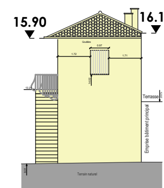
FAÇADE NORD - GARDIEN
