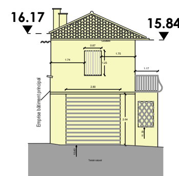
FAÇADE SUD - GARDIEN
