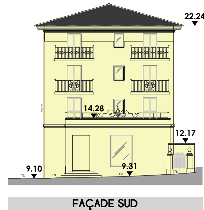
FAÇADE SUD
