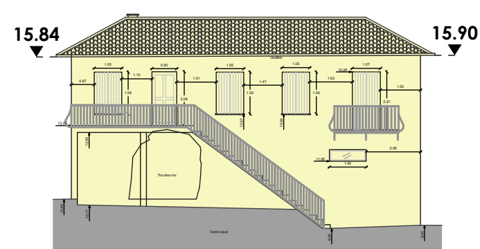
FAÇADE EST - GARDIEN
