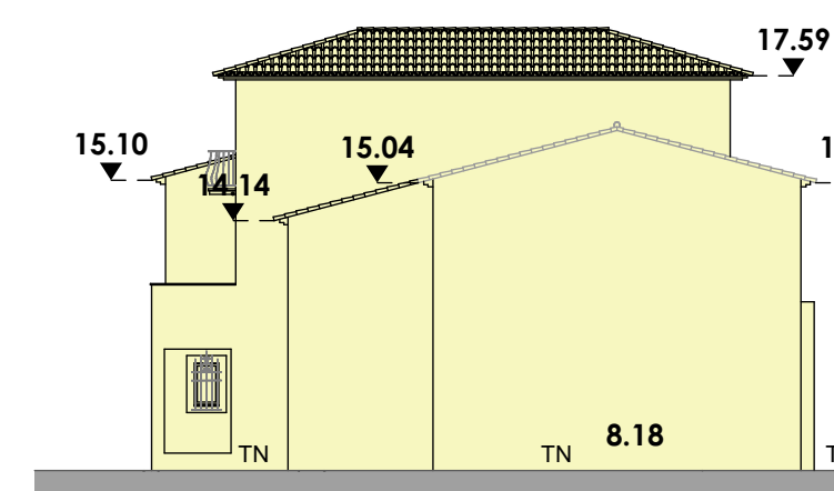
FAÇADE EST - VILLA
