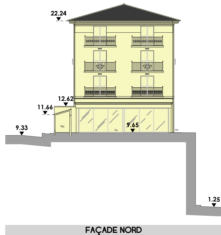
FAÇADE NORD
