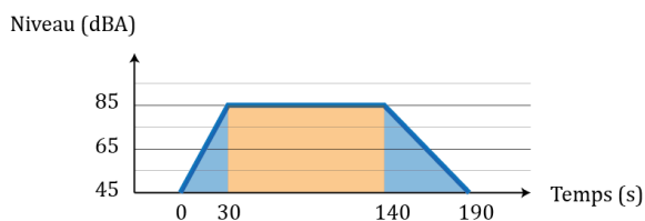
Figure 9 : Schéma des niveaux en dBA du EC130 à 30 m du point de pose
