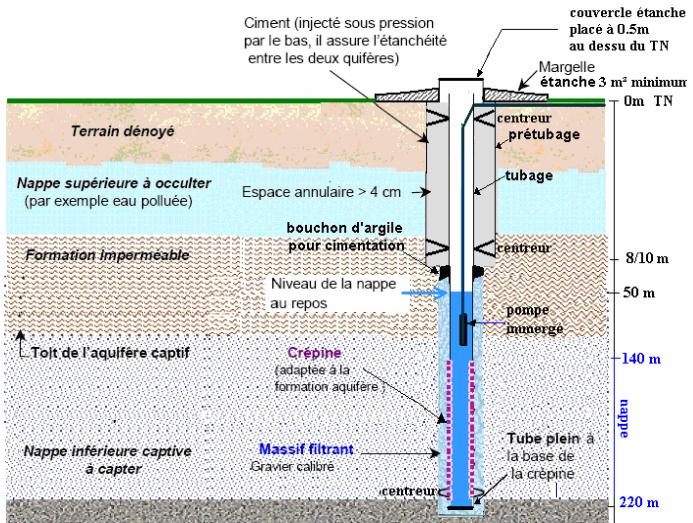
Coupe prévisionnelle du forage projeté faisant office de plan du projet
