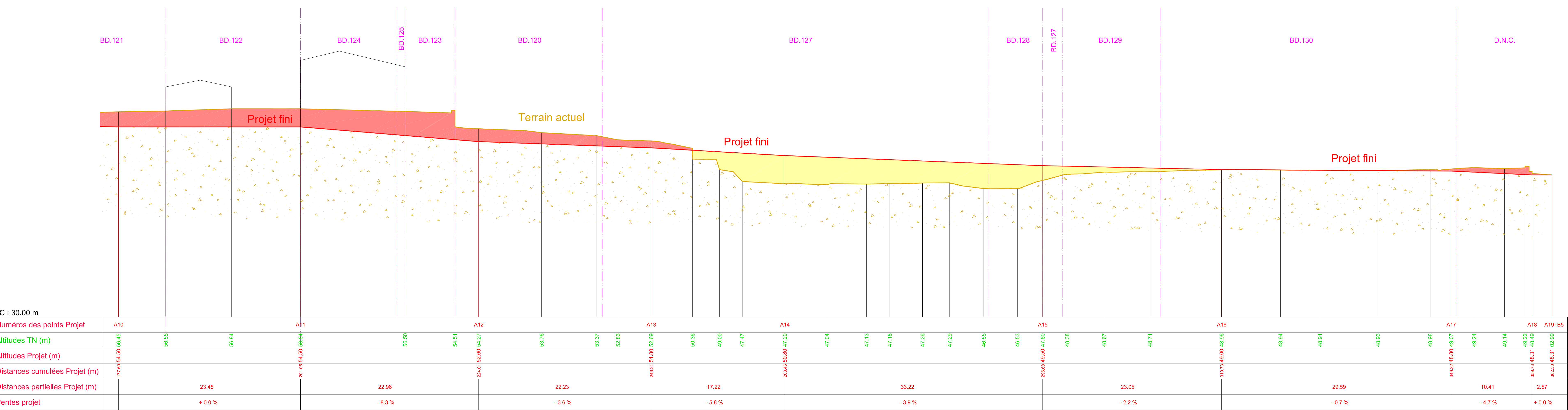
PROFIL EN LONG : AXE A10-A19
