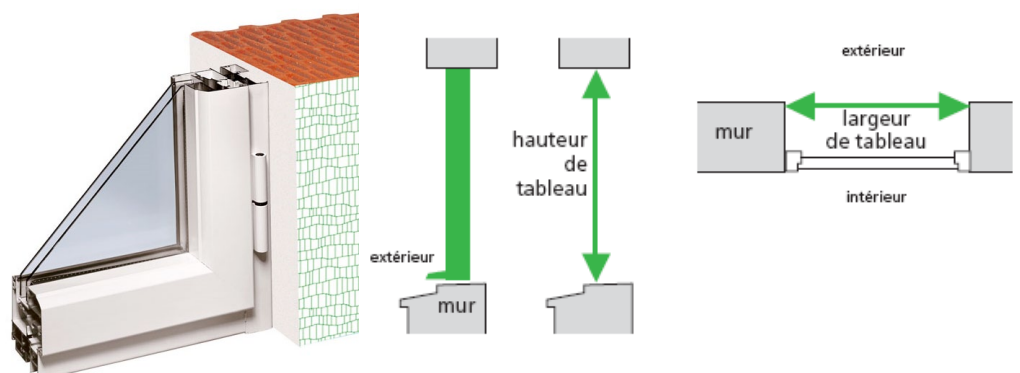
Figure 6 : schéma de la pose en tunnel
