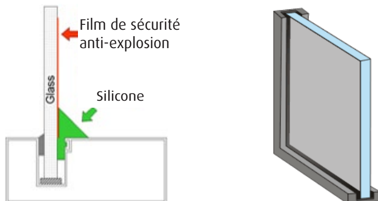
Figure 11 : fixation chimique du film
