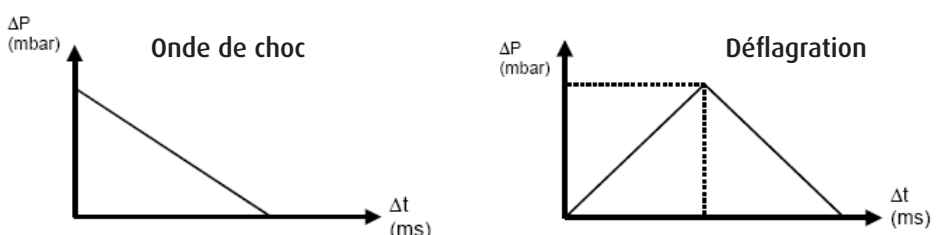
Figure 15 : Signaux de surpression typiques
