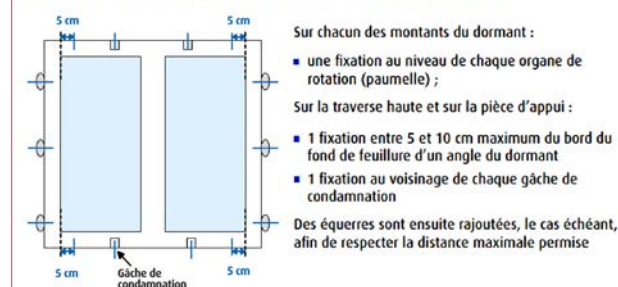
Figure 2 : disposition des fixations principales pour les fenêtres à ouverture à la française avec système de fermeture à renvoi d'angle en face 1 à 4 d'une construction dans la zone 20-50 mbar
