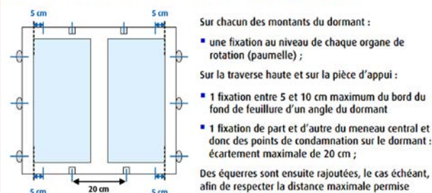
Figure 1 : disposition des fixations principales pour les fenêtres à ouverture à la française à deux vantaux munies d'un système de fermeture à sortie de tringle en face 1 à 4 d'une construction dans la zone 20-50 mbar
