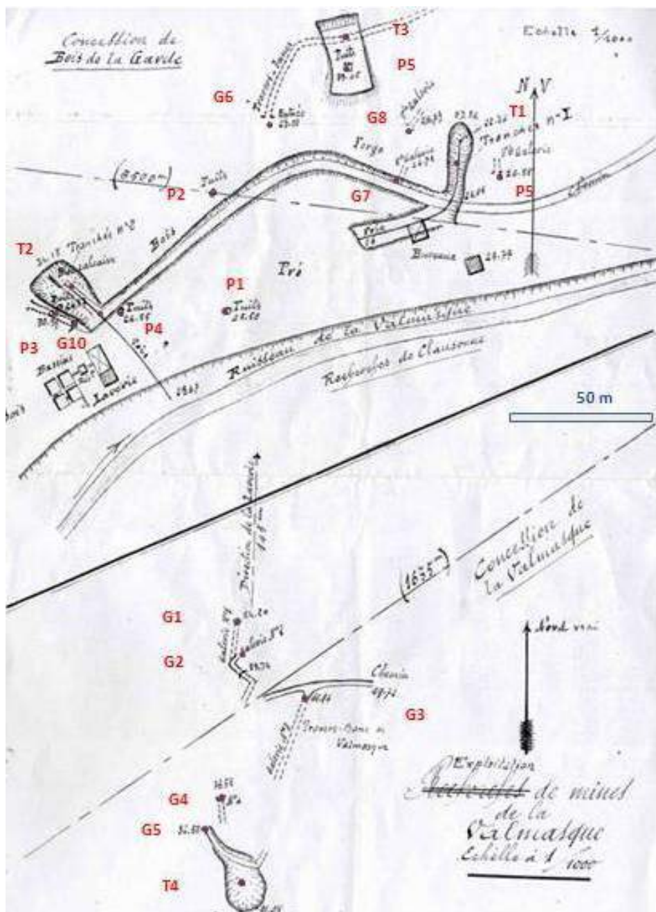
Figure 10 – Détail des travaux du site de Clausonnes (carte décalée au sud).
