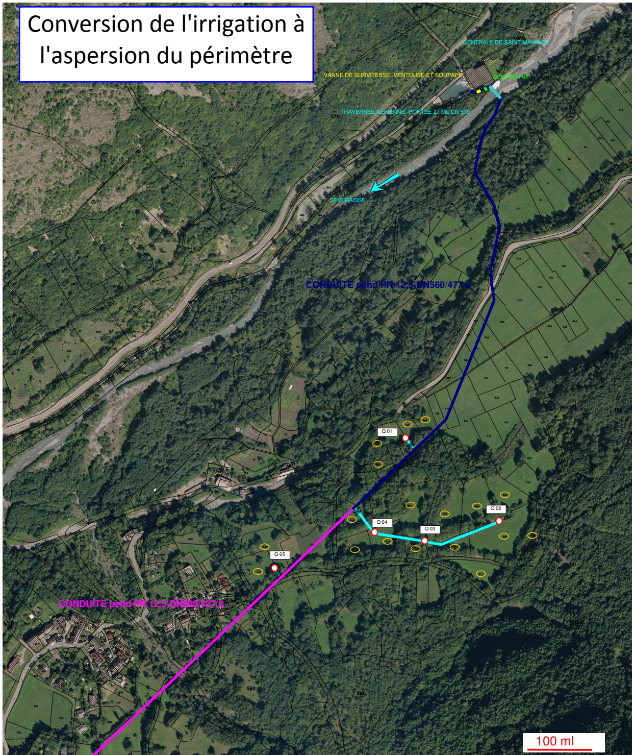
PLAN 2 - PARCELLAIRE 1 - ADDUCTION PARTIE AMONT
