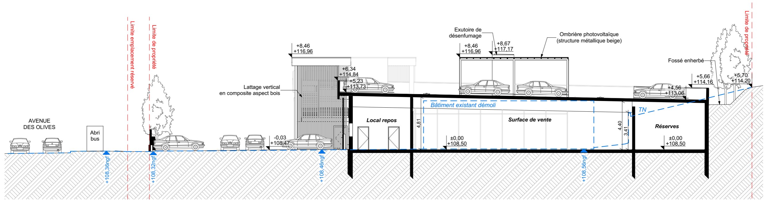
Coupe AA - Echelle : 1/200e
