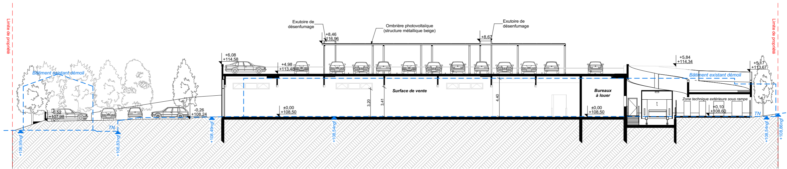
Coupe BB - Echelle : 1/250e
