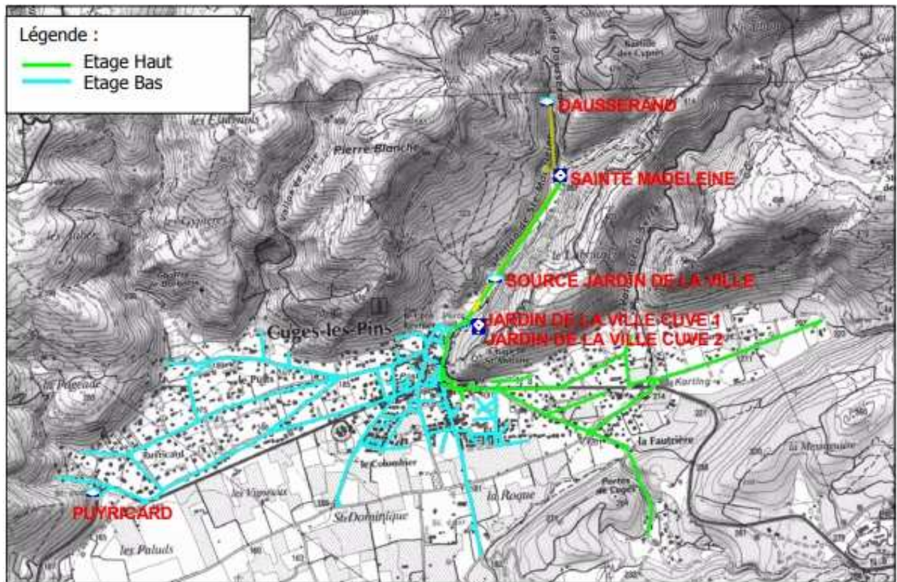
Réseau d'eau potable de la ville de Cuges (terrain hors desserte)
