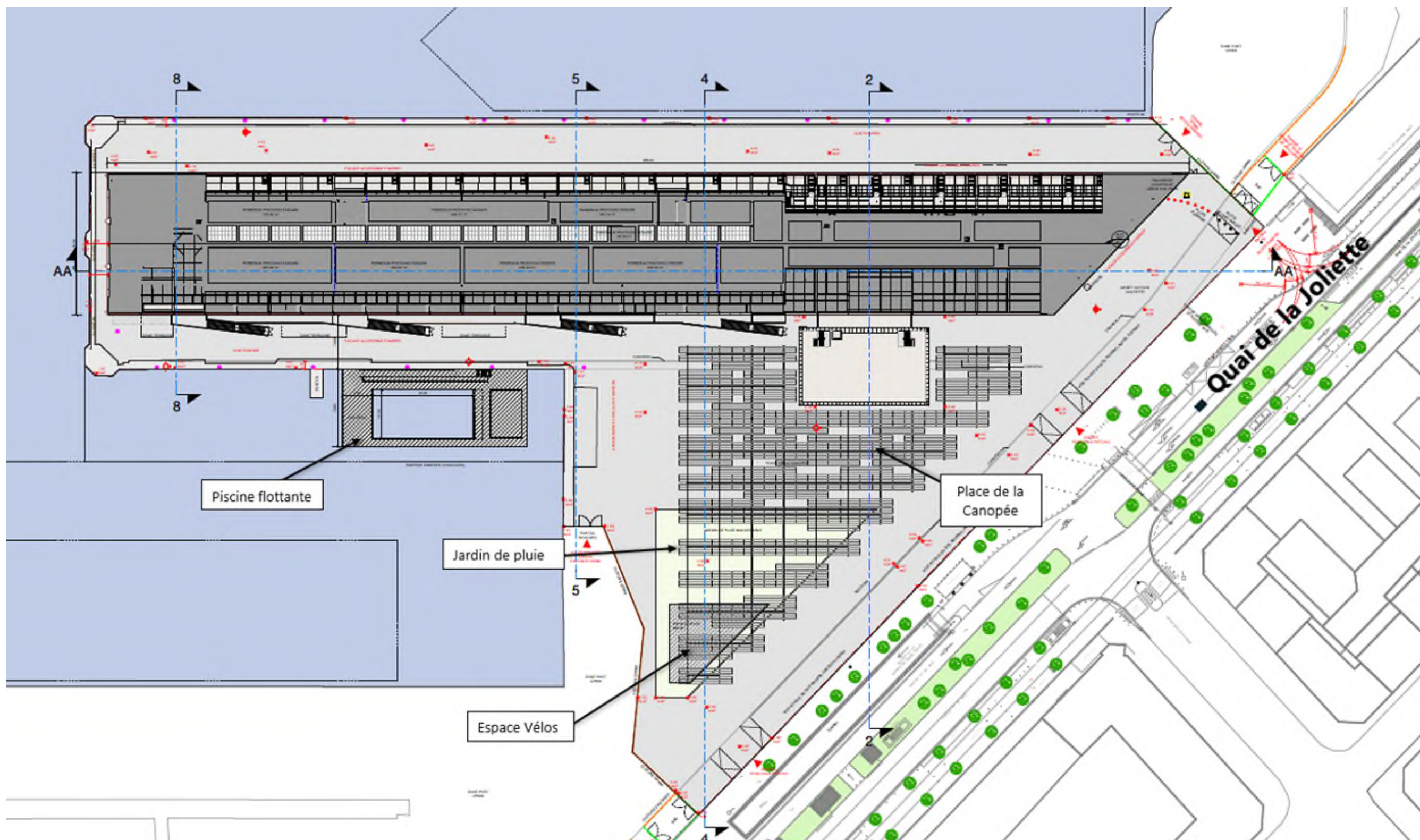
Figure 2 - Plan de masse général du projet – stade concours (ADIM Provence)
