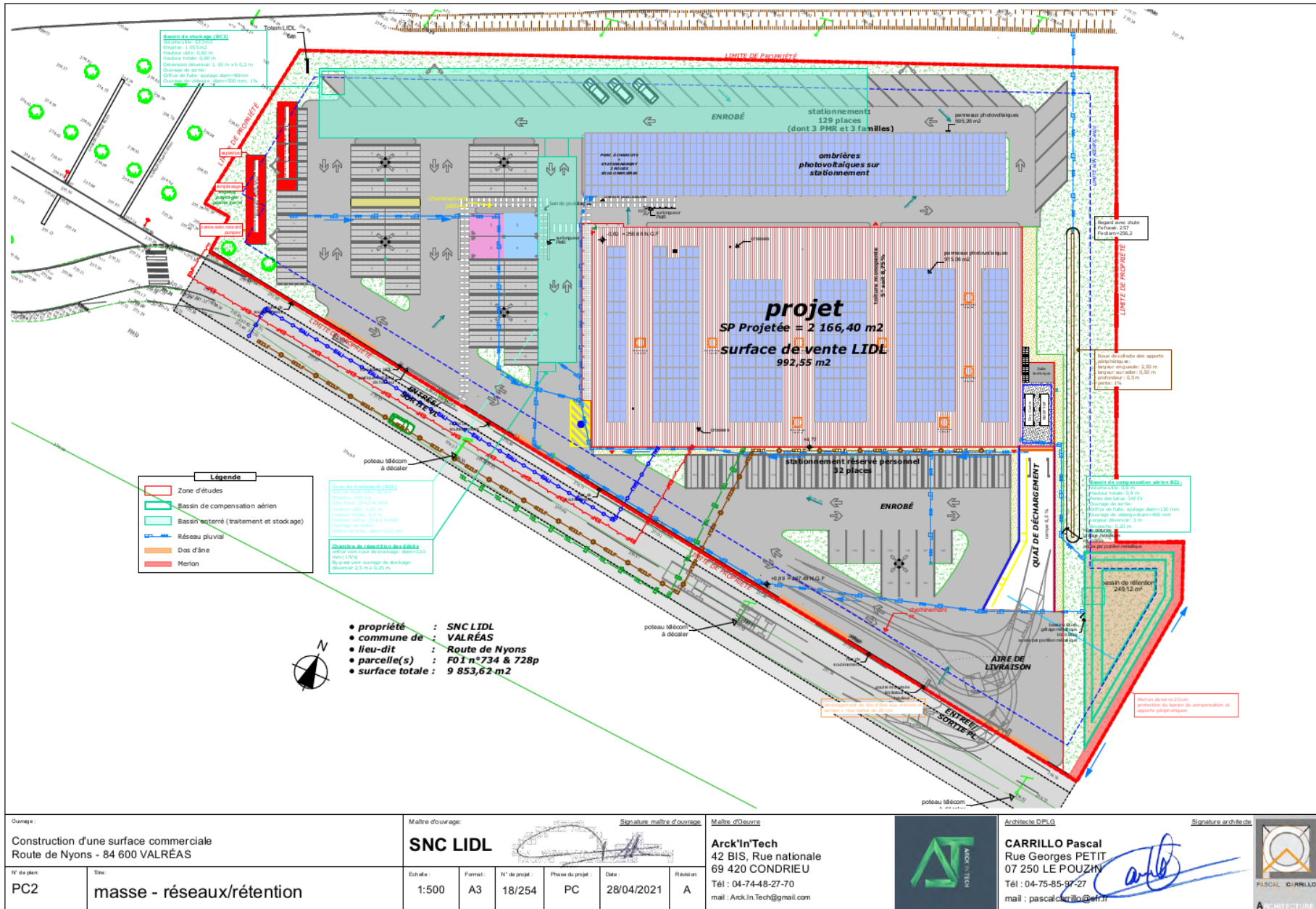
Illustration 3 : Principes d'assainissement pluvial retenus (extrait du PC)
