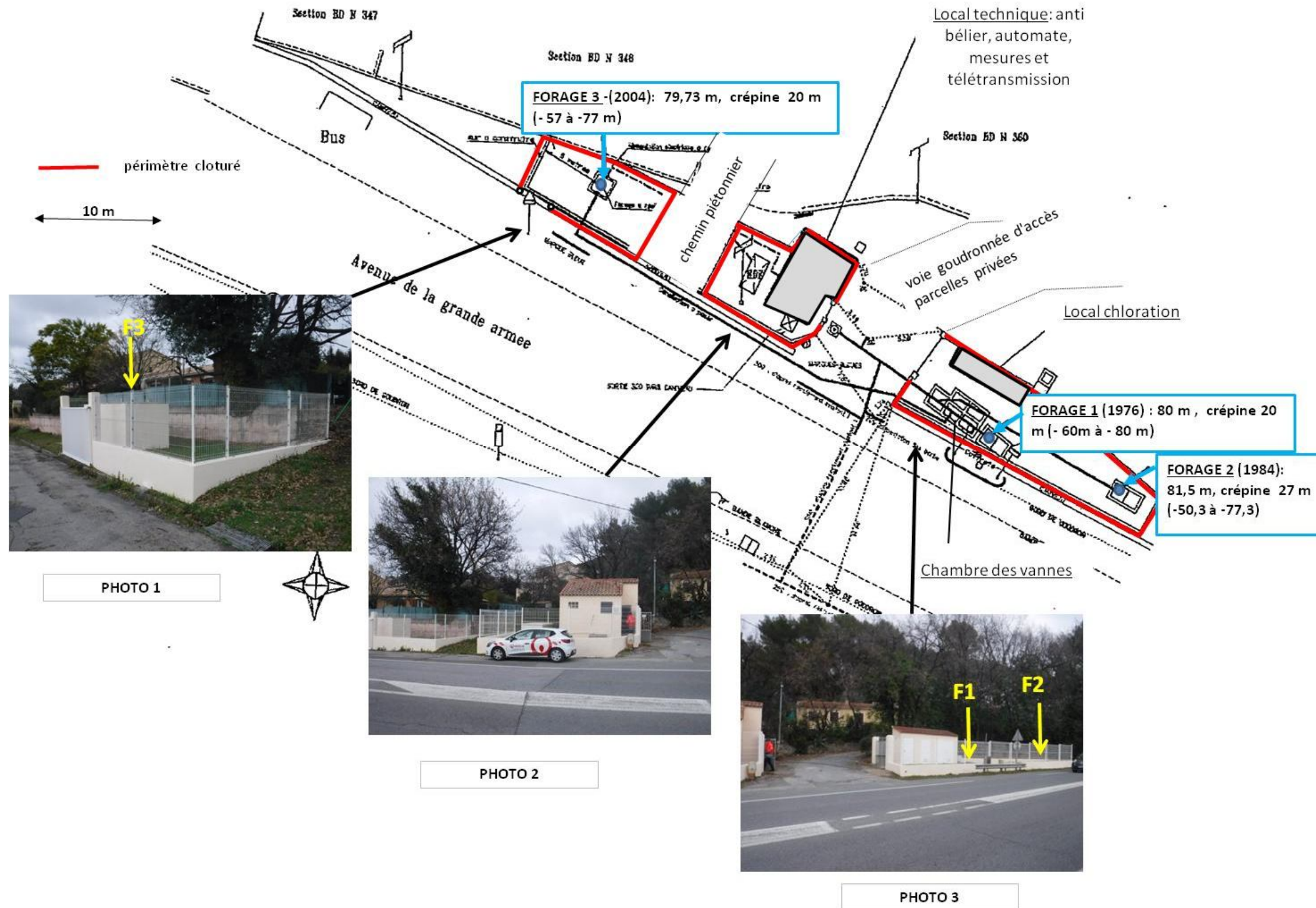
Figure 1: Plans et vues des installations présentes sur le captage Sainte Anne
