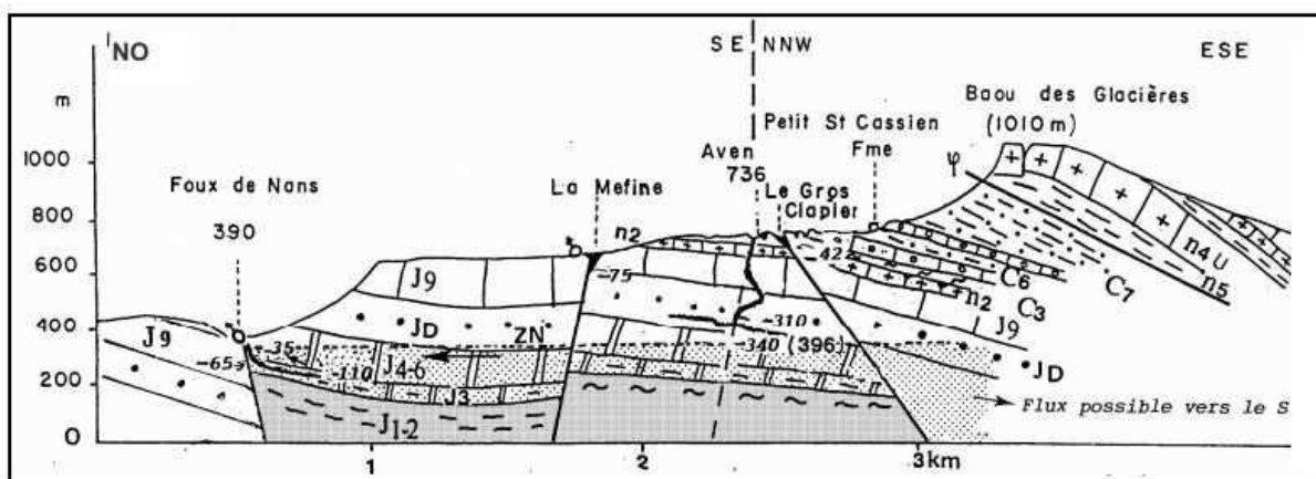
Figure 1 : coupe du Baou des Glacières à la Grande Foux de Nans-les-Pins, montrant la position et le fonctionnement de son aquifère (M. JULIAN et J. NICOD, 1989, modifiée).
