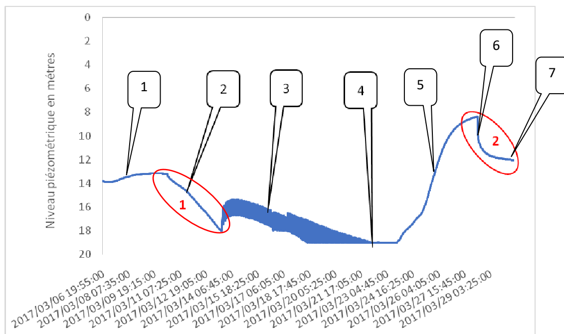
Figure 2: Variation du niveau piézométrique du forage Rondoline durant toute la période du test
