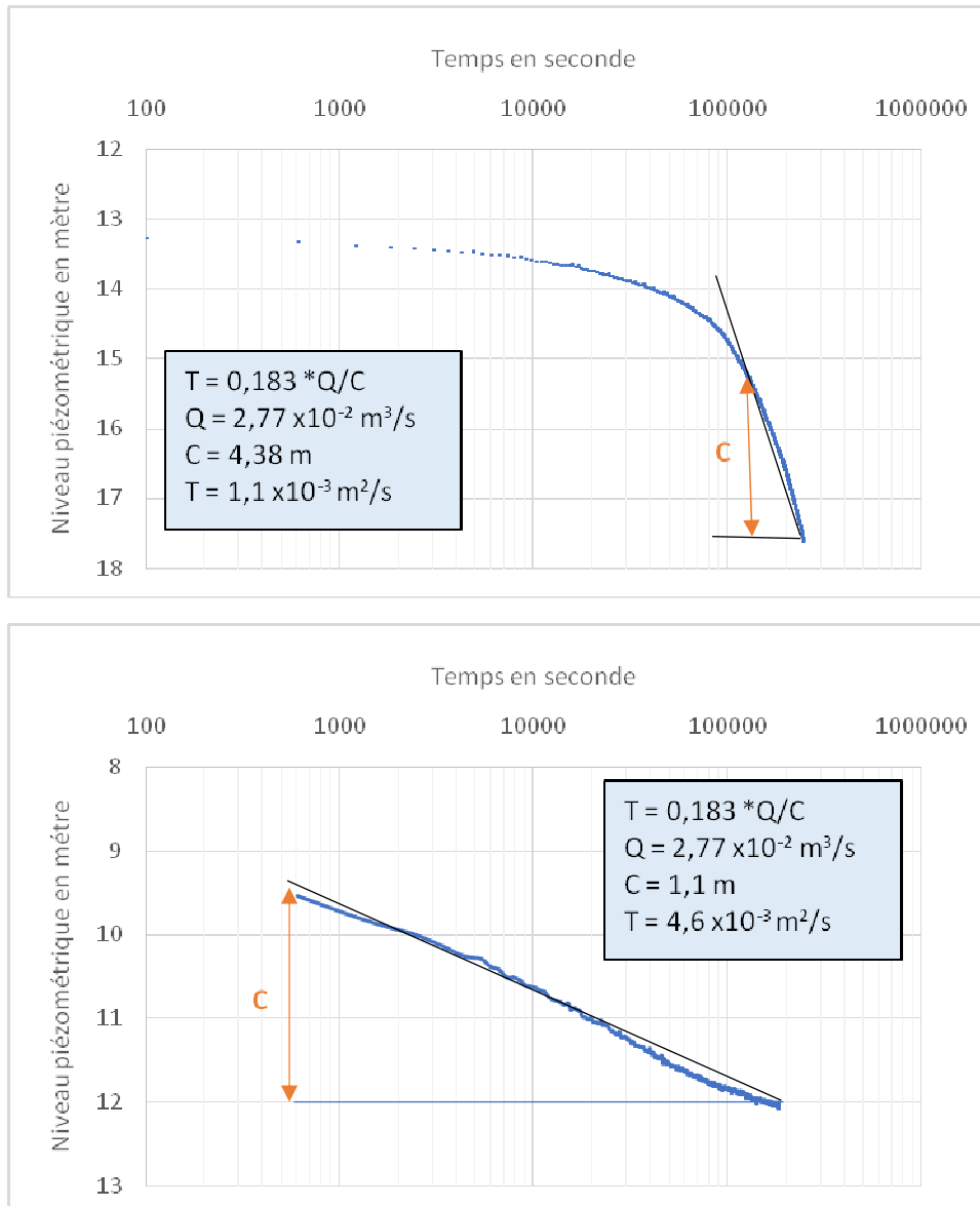
Figure 3: courbe de rabattement du forage durant deux pompages de longue durée
