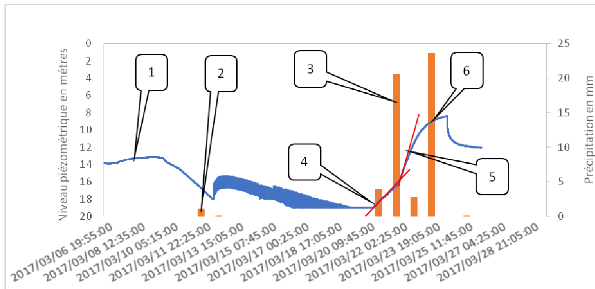
Figure 4: Evolution du niveau piézométrique et hauteur de précipitations
