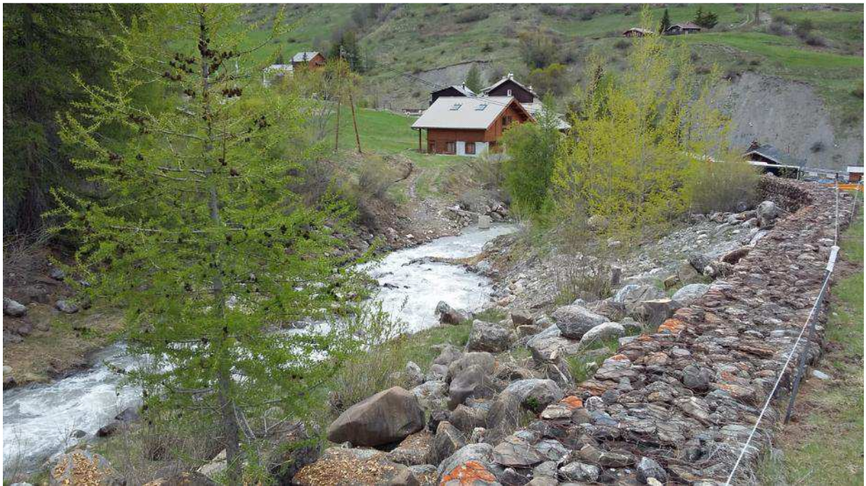
Tronçon intermédiaire aval (vue vers aval) – tranche 3 de travaux : partie aval de la digue de protection avec gabions en crête, le long du parking
