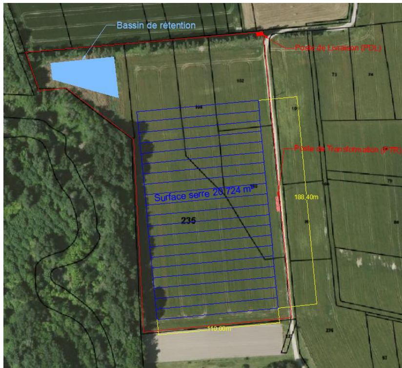
Figure 2 – Implantation du projet – Source REDEN Solar
