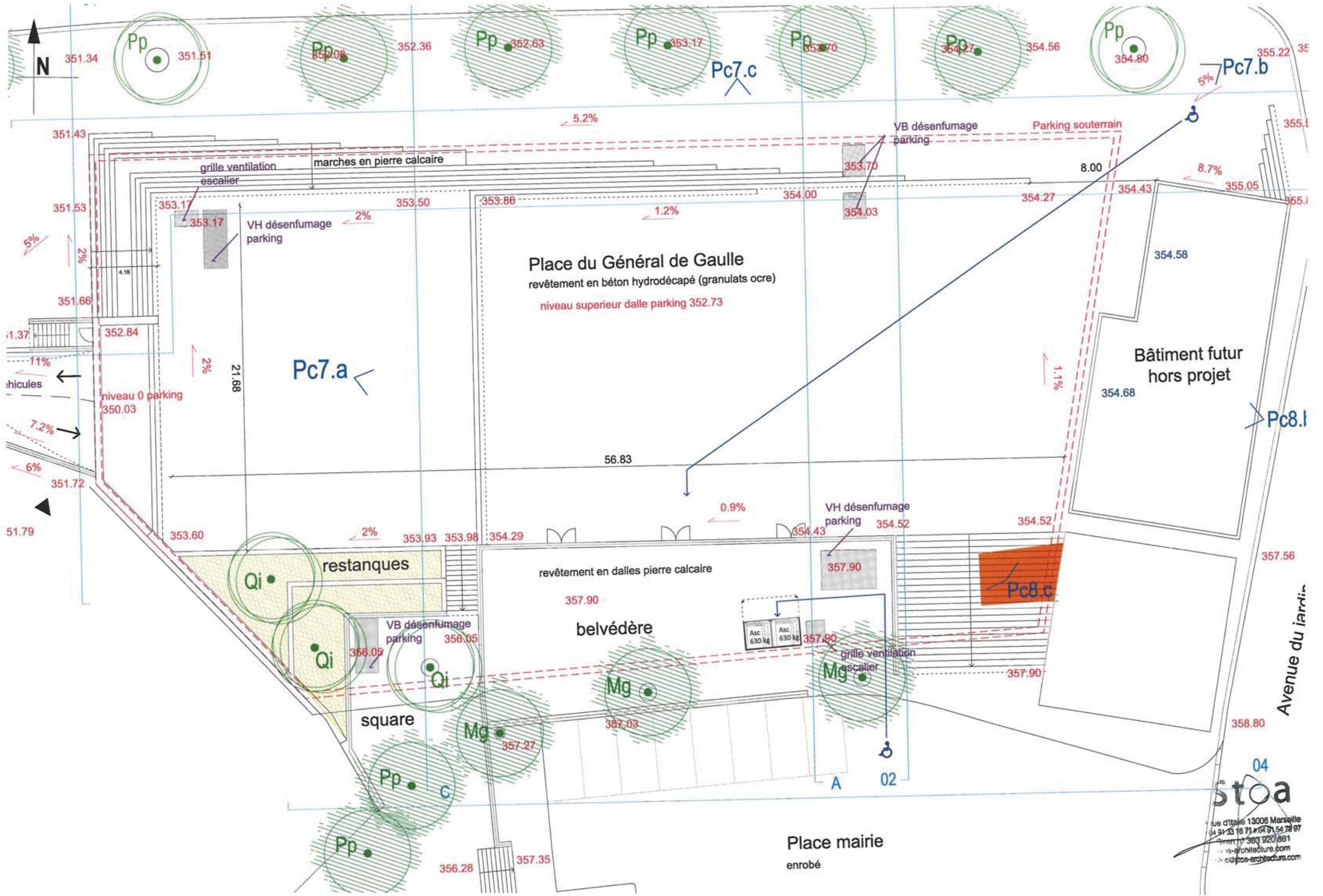
8.1.4/ Plan du projet place haute (place de la mairie)
