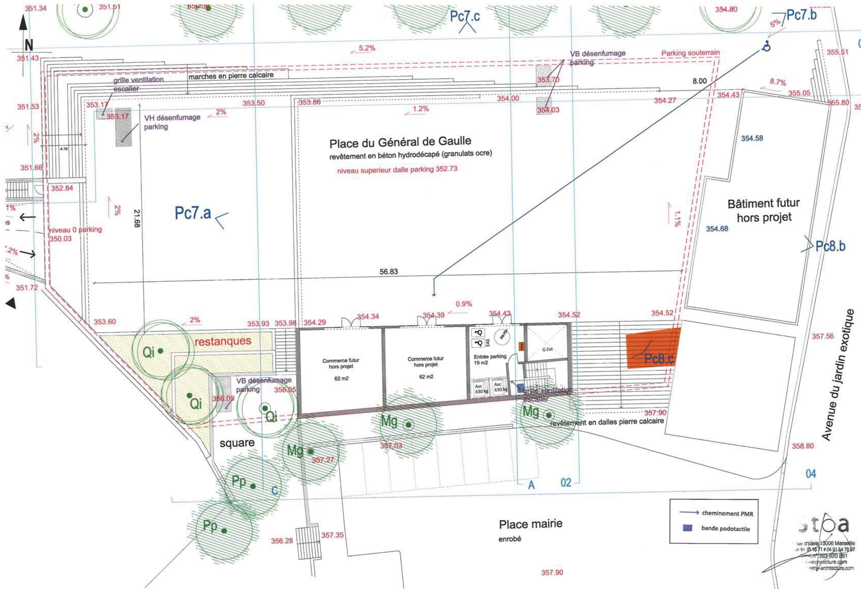
8.1.4/ Plan du projet place basse (commerces)
