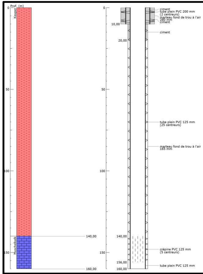
Coupe prévisionnelle forage F2
