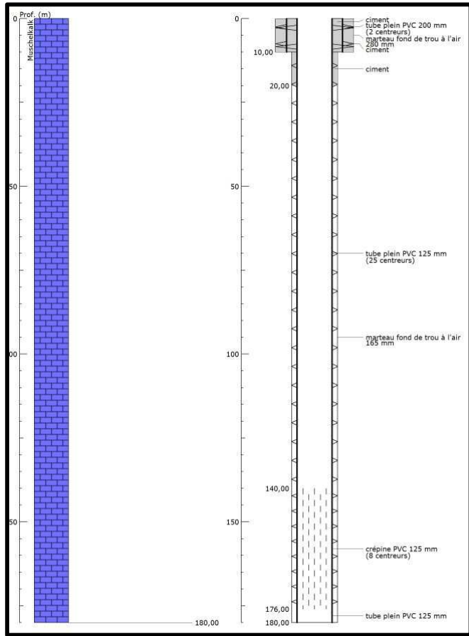
Coupe prévisionnelle forage F1
