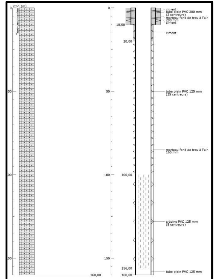
Coupe prévisionnelle forages F3
