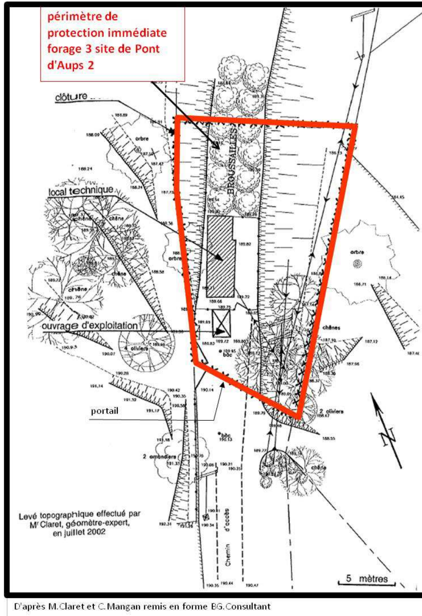
Figure 2: Détail du champ captant et du périmètre de protection immédiate du site Pont d'Aups 2.
