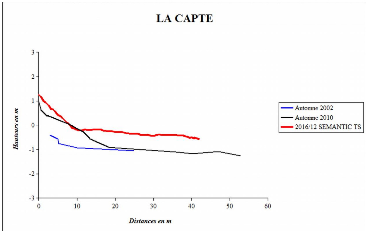
Figure 9 : Coupes des profils bathymétriques – plage de La Capte
