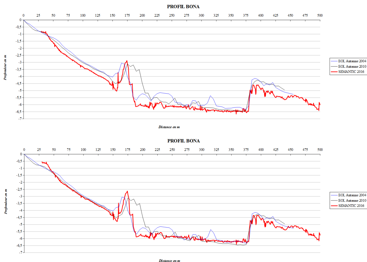
Figure 7 : Coupes des profils bathymétriques – plage de Bona – Avec les données 2016 en NGF (haut) et en cote marine (bas)
