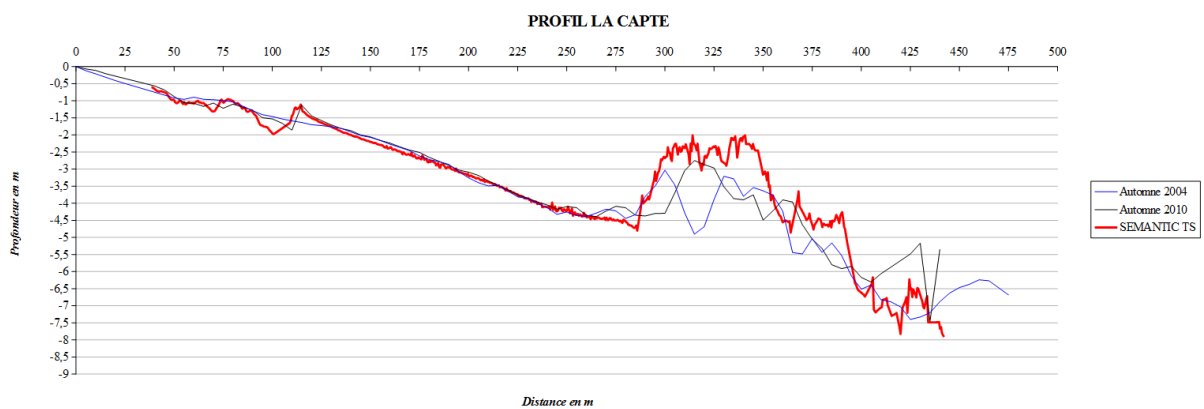
Figure 8 : Coupes des profils bathymétriques – plage de La Capte
