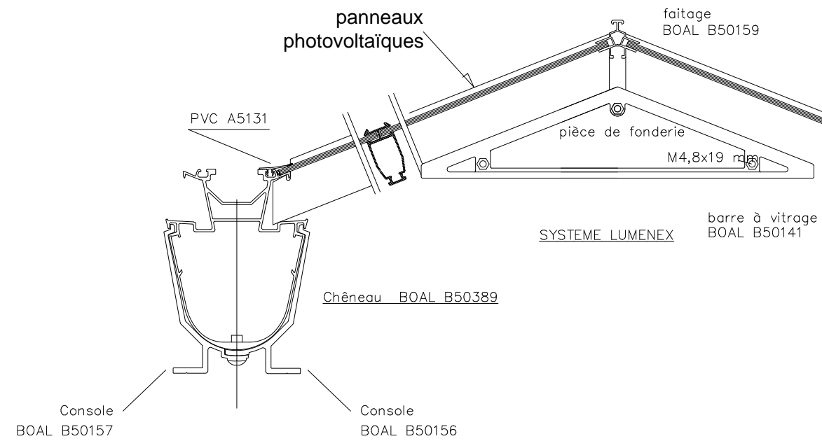
Détail de principe toiture (Détail du fabricant de serres) sans échelle
