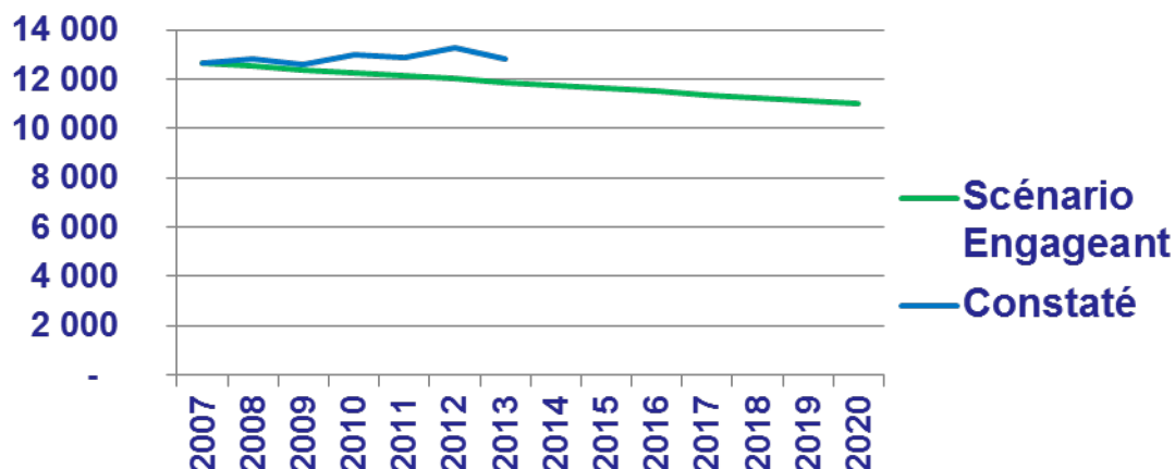
Consommation totale d'énergie finale (en ktep)
