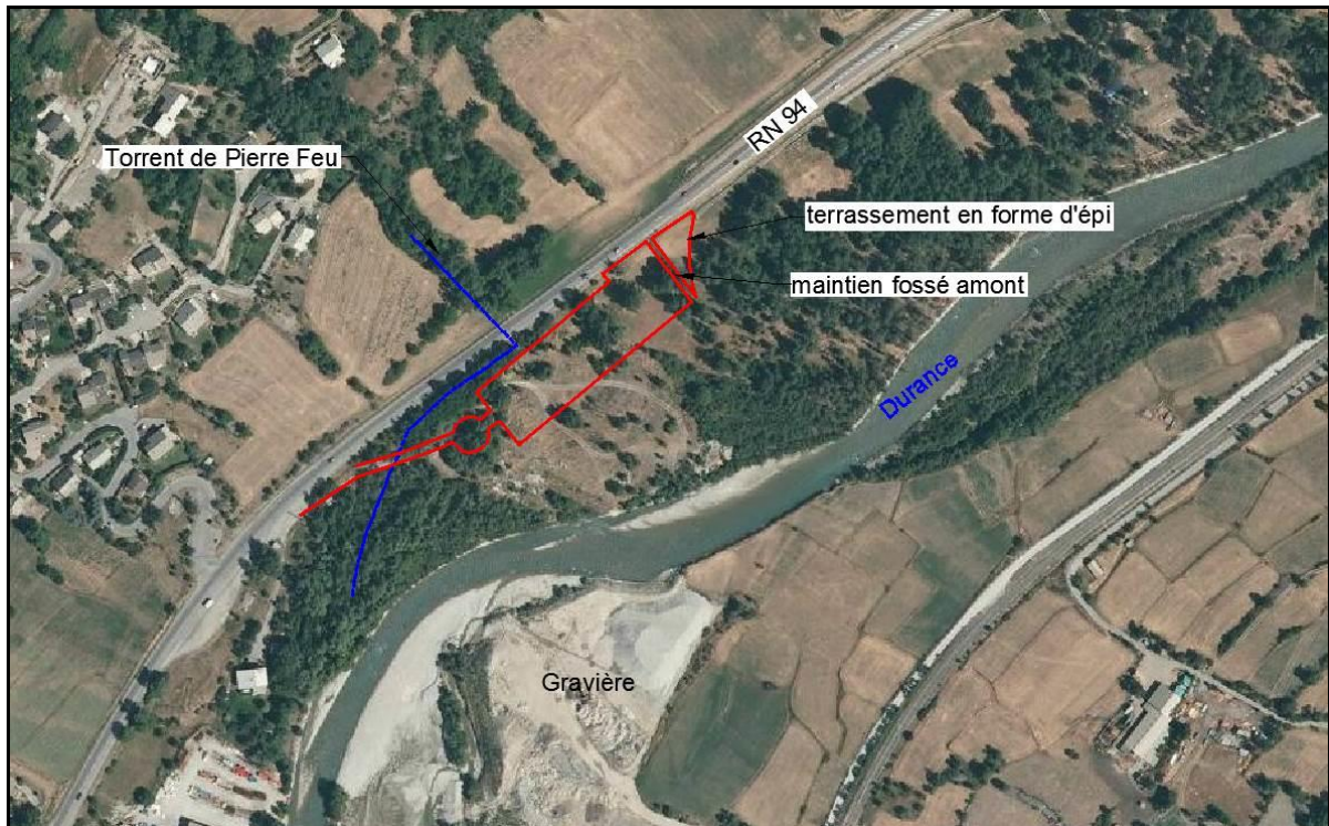
Figure 18 : proposition d'implantation de la plateforme
