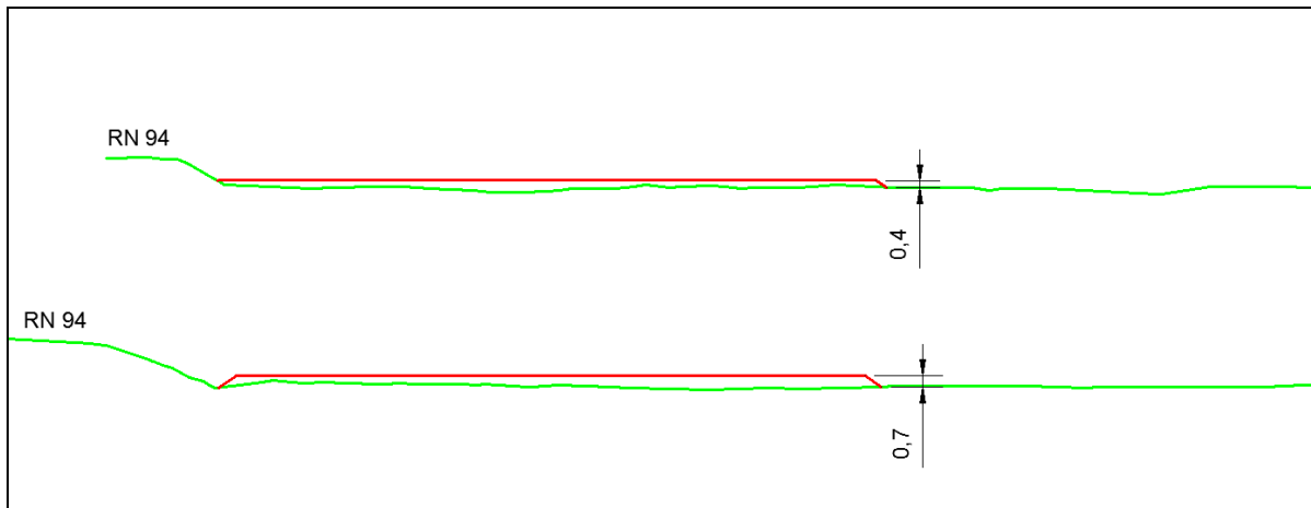
Figure 19 : illustration des coupes type en amont (en haut) et aval (en bas) de la plateforme
