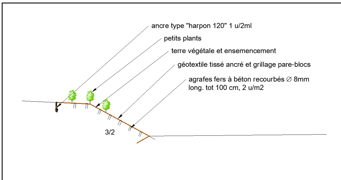
Figure 21 : principe de confortement du talus de la plateforme
