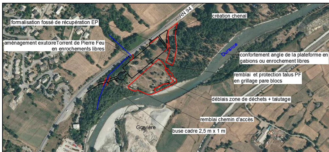
Figure 20 : illustration des aménagements hydrauliques proposés
