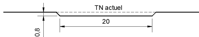
Figure 23 : coupe schématique chenal amont
