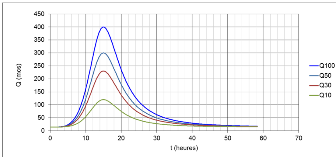
Figure 9 : hydrogrammes de crue
