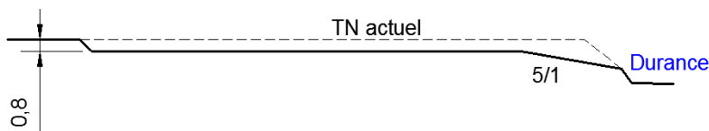
Figure 22 : coupe schématique déblais et talutage
