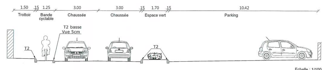
COUPE D-D
