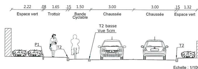
COUPE E-E
