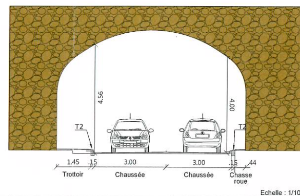
COUPE E-E
