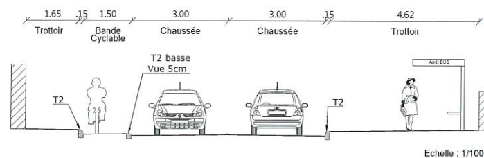
COUPE B-B
