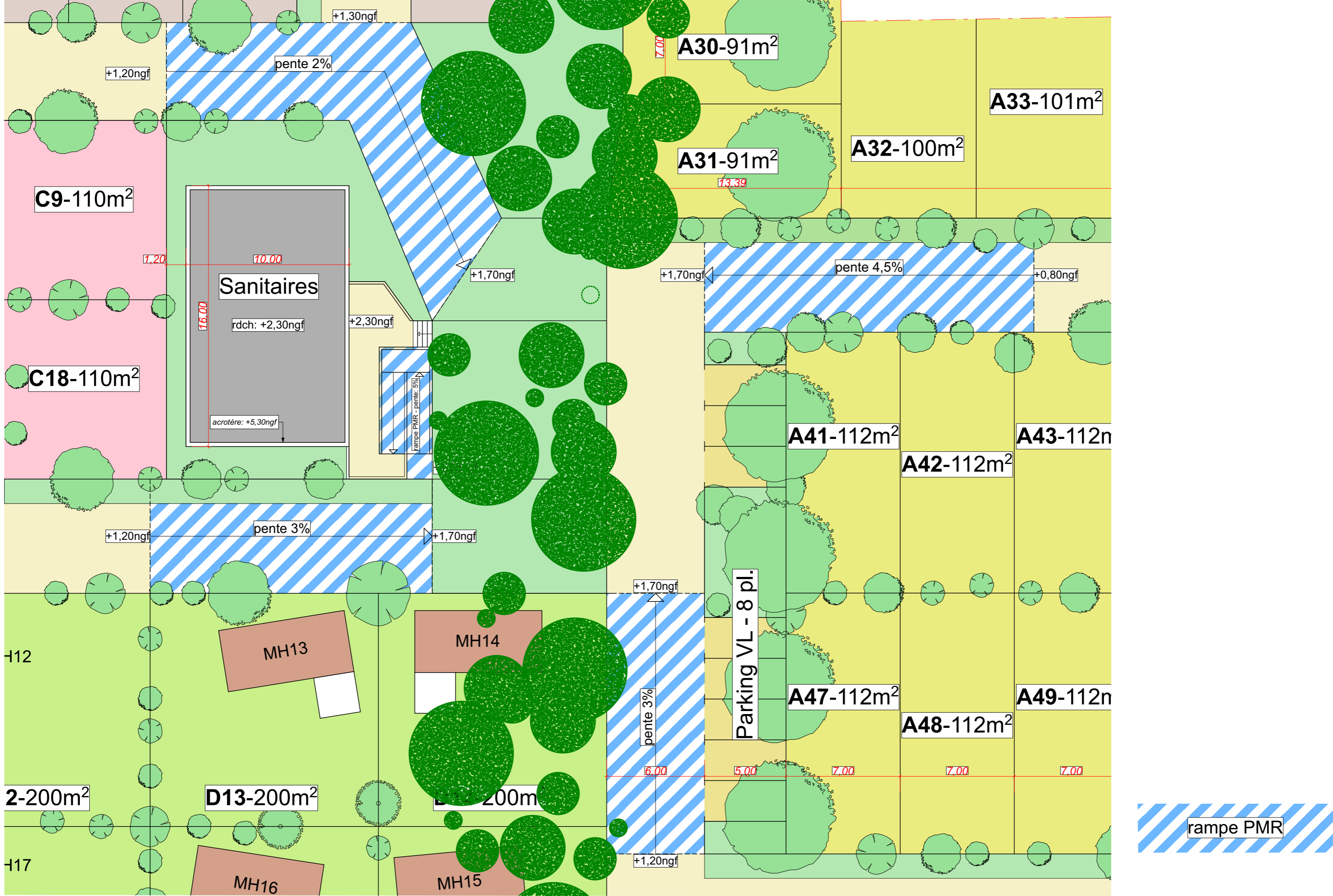
Implantation des rampes d'accès PMR au bâtiment sanitaires communs - éch: 1/200e
