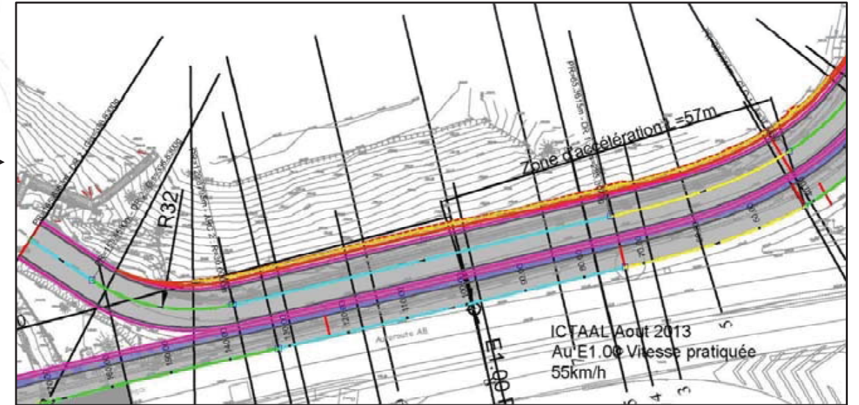
Aménagement de la bretelle d'insertion et de la RD
