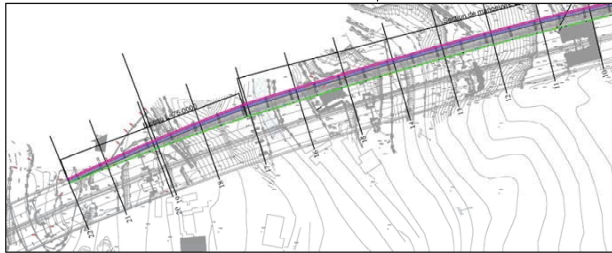
Aménagement du viaduc
