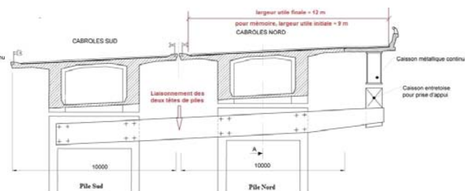
Coupe de principe de l'élargissement du tablier
