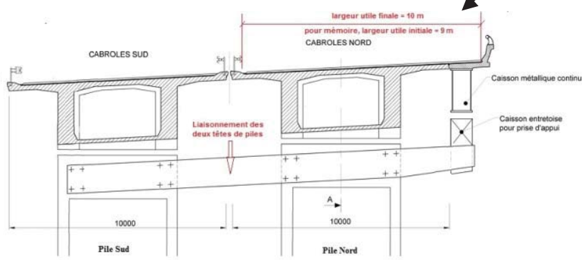
Coupe intermédiaire de principe du biseau
