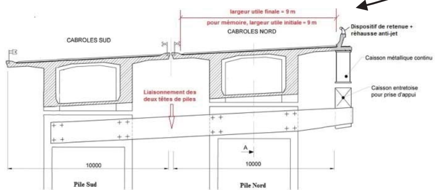
Coupe terminale de principe du biseau
