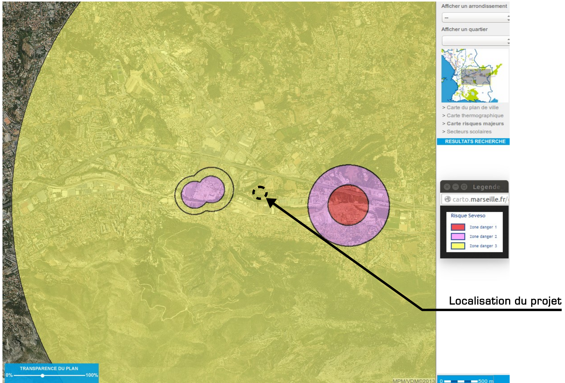
Identification du risque industriel mesuré au niveau de la zone d'étude où s'insère le projet - Source : carto.marseille-provence.fr
