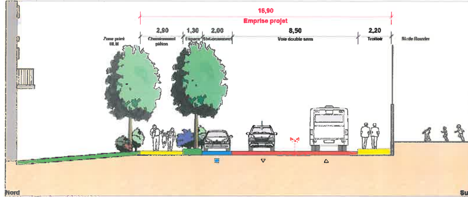
COUPE AA' ETAT DES LIEUX
