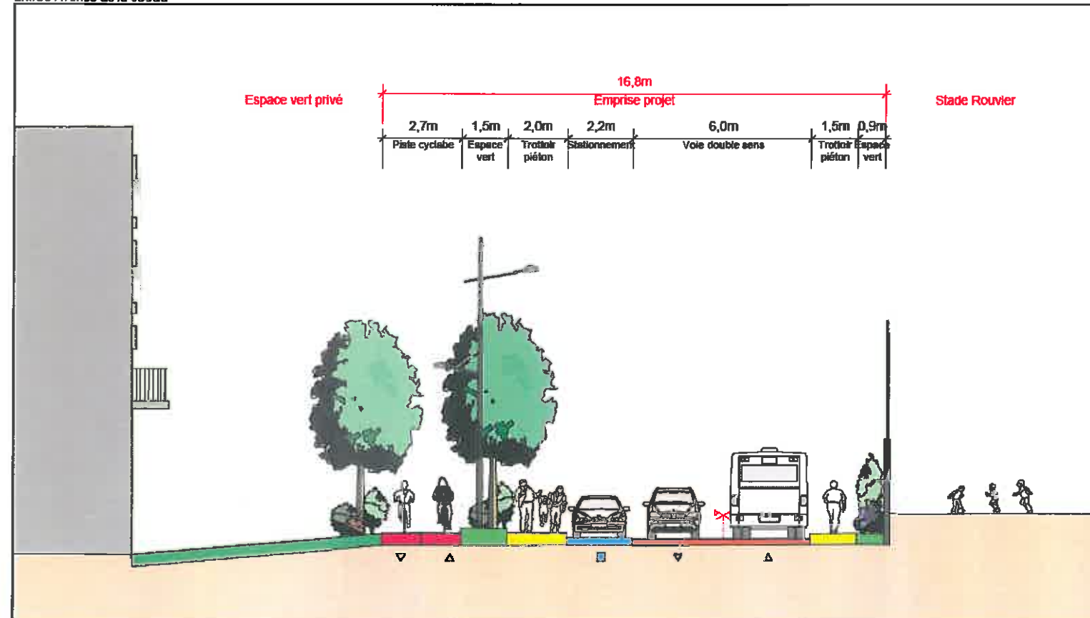
Coupe AA' Entrée Avenue de la Soude
